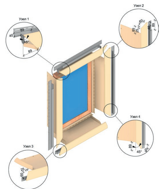
Рис. 18 Обрамление оконного проёма при помощи универсального околооконного профиля 89/254 мм с J-профилем 16 мм.
