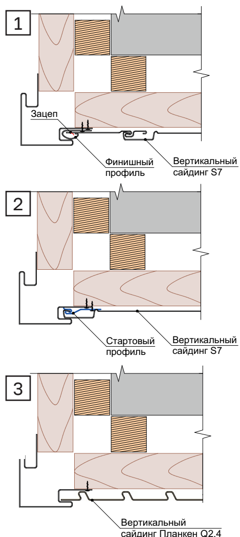
Рис. 30 Оформление подхода вертикального сайдинга Döcke тонкой частью к вертикальным профилям.
