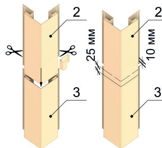
Рис. 8 Подрезка и стыковка наружных углов.
