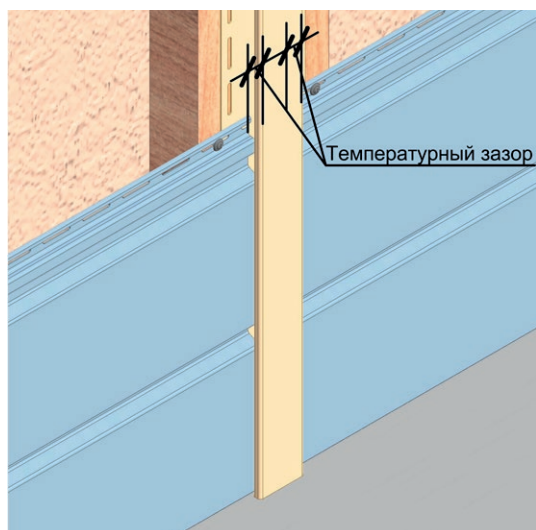
Рис. 23 Стыковка панелей горизонтального сайдинга Döcke через Н-профиль.
