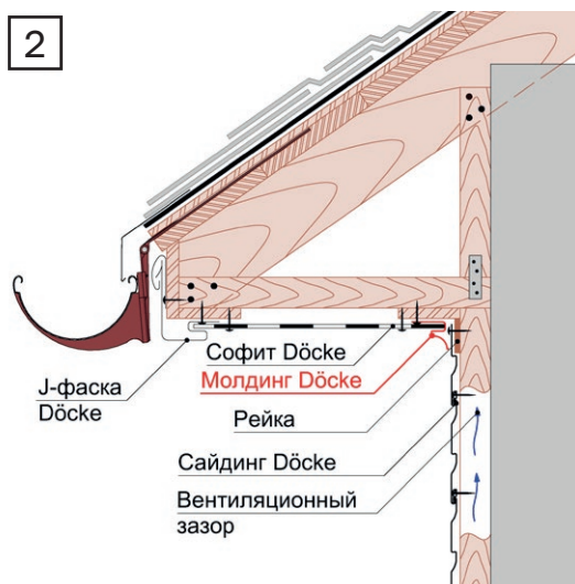
Рис. 27 Присыкание сайдинга Döcke к карнизному свесу при помощи молдинга.
