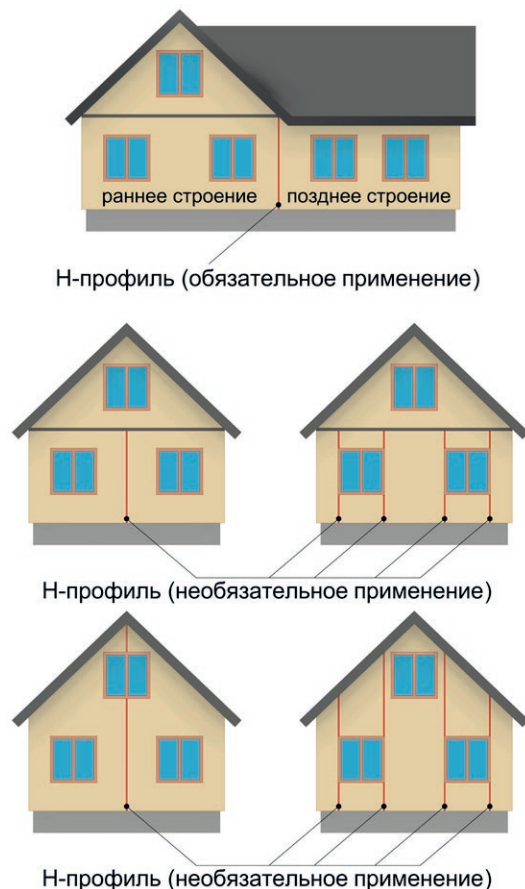
Рис. 11 Применение Н-профиля.
