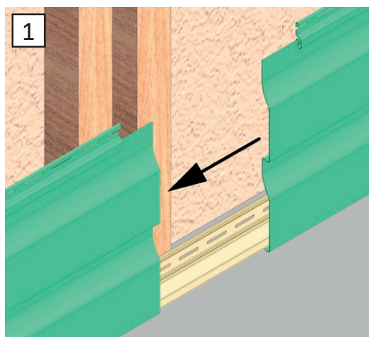
Рис. 23 Стыковка панелей горизонтального сайдинга Döcke через Н-профиль.
