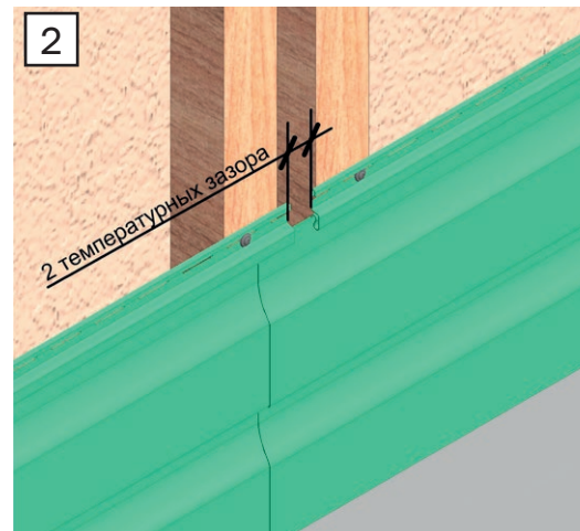
Рис. 24 Стыковка панелей горизонтального сайдинга Döcke внахлест.
