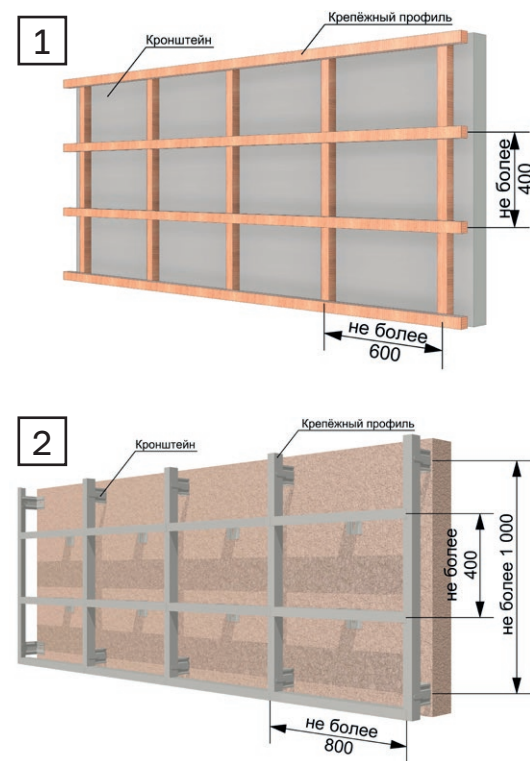
Рис. 28 Деревянная и металлическая обрешётка под вертикальный сайдинг Döcke.
