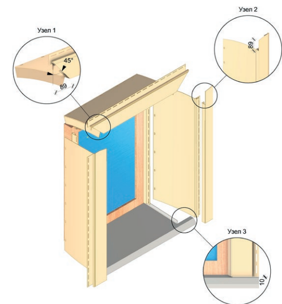
Рис. 20 Обрамление оконного проёма при помощи наличника 89 мм с откосом 254 мм.
