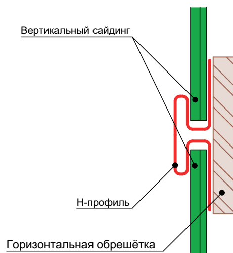
Рис. 31 Стыковка вертикального сайдинга по длине.
