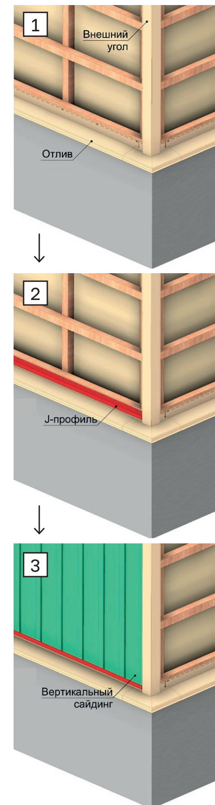
Рис. 29 Подготовка к монтажу вертикального сайдинга Döcke.
