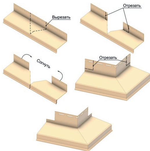
Рис. 4 Изготовление внешнего углового элемента отлива Döcke.
