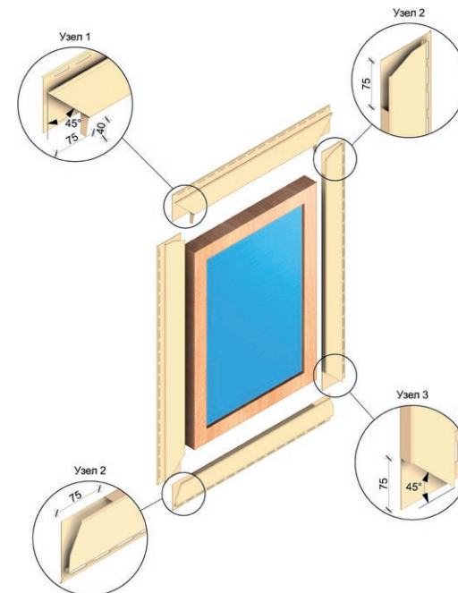
Рис. 13 Обрамление оконного проёма при помощи наличника 75 мм.
