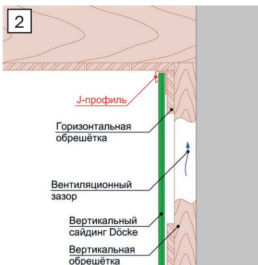
Рис. 37 Устройство примыканий к горизонтальным поверхностям и окончание монтажа панелей вертикального сайдинга на стене.
