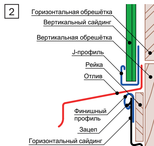
Рис. 32 Стыковка горизонтального сайдинга с вертикальным в случае, когда горизонтальный сайдинг снизу, а вертикальный сверху.
