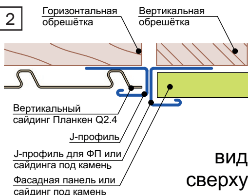
Рис. 36 Вертикальная стыковка горизонтального и вертикального сайдинга с фасадными панелями или сайдингом под камень.
