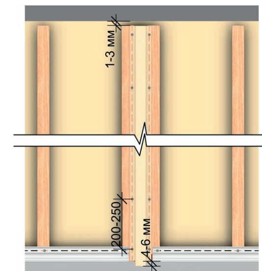
Рис. 10 Установка Н-профиля.
