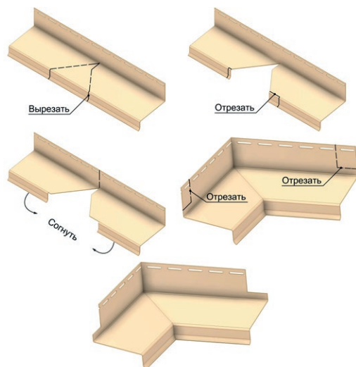
Рис. 6 Изготовление внутреннего углового элемента отлива Döcke.
