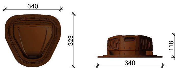
Геометрические размеры
