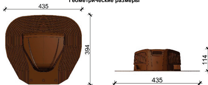
Геометрические размеры
